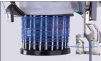
Bobine d'enroulement à séparation
